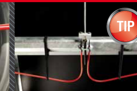
Držáky lanovodů AL-KO zabraňují vnikání vody a zamrzání lanovodů.
